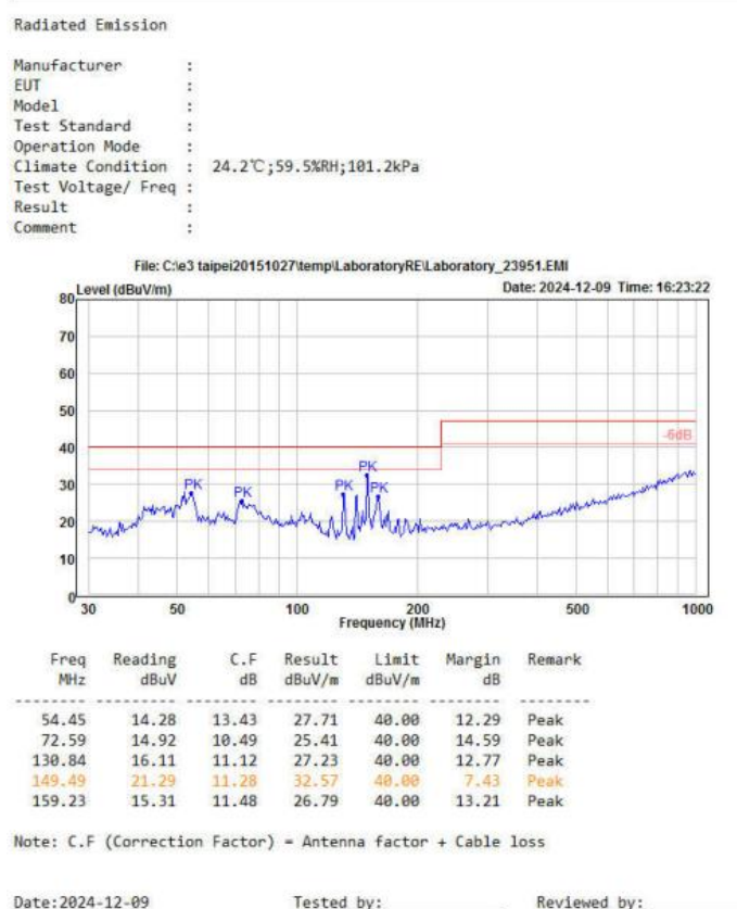
图 6-7 辐射测试垂直方向
