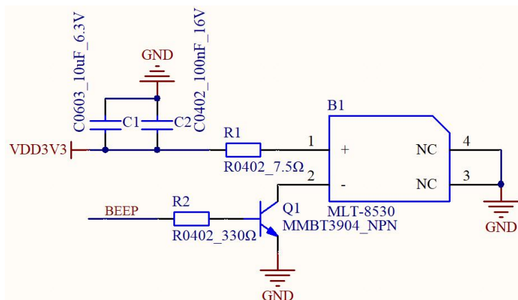
图 2-2 蜂鸣器电路示意
