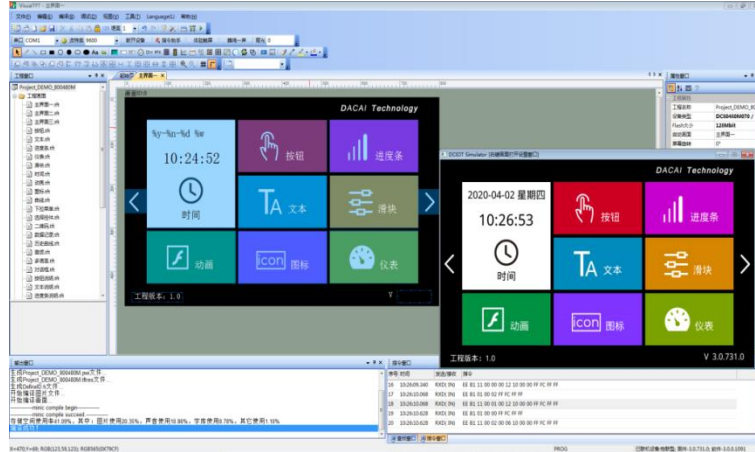
图 8-1 VisualTFT 主界面
